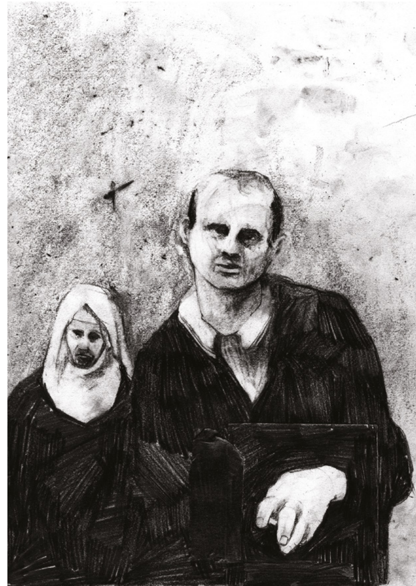
Behave
